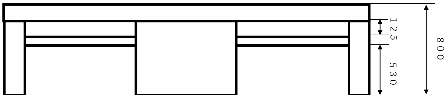
実験台正面図
