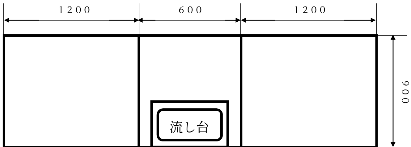
実験台平面図
